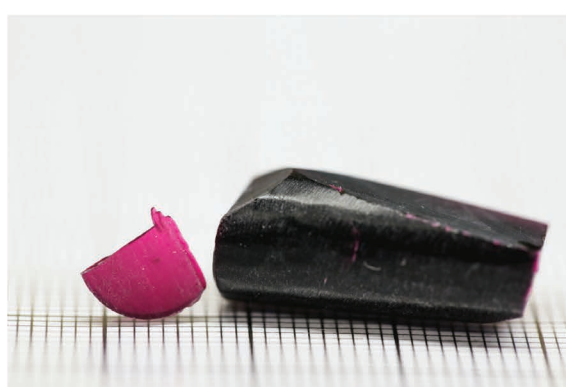
\text{NaSrCo}_2\text{F}_7
